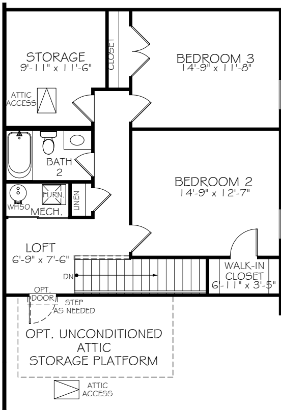
OPT. SECOND FLOOR - 2 BEDROOM/ 1 BATH (OPT.A)
